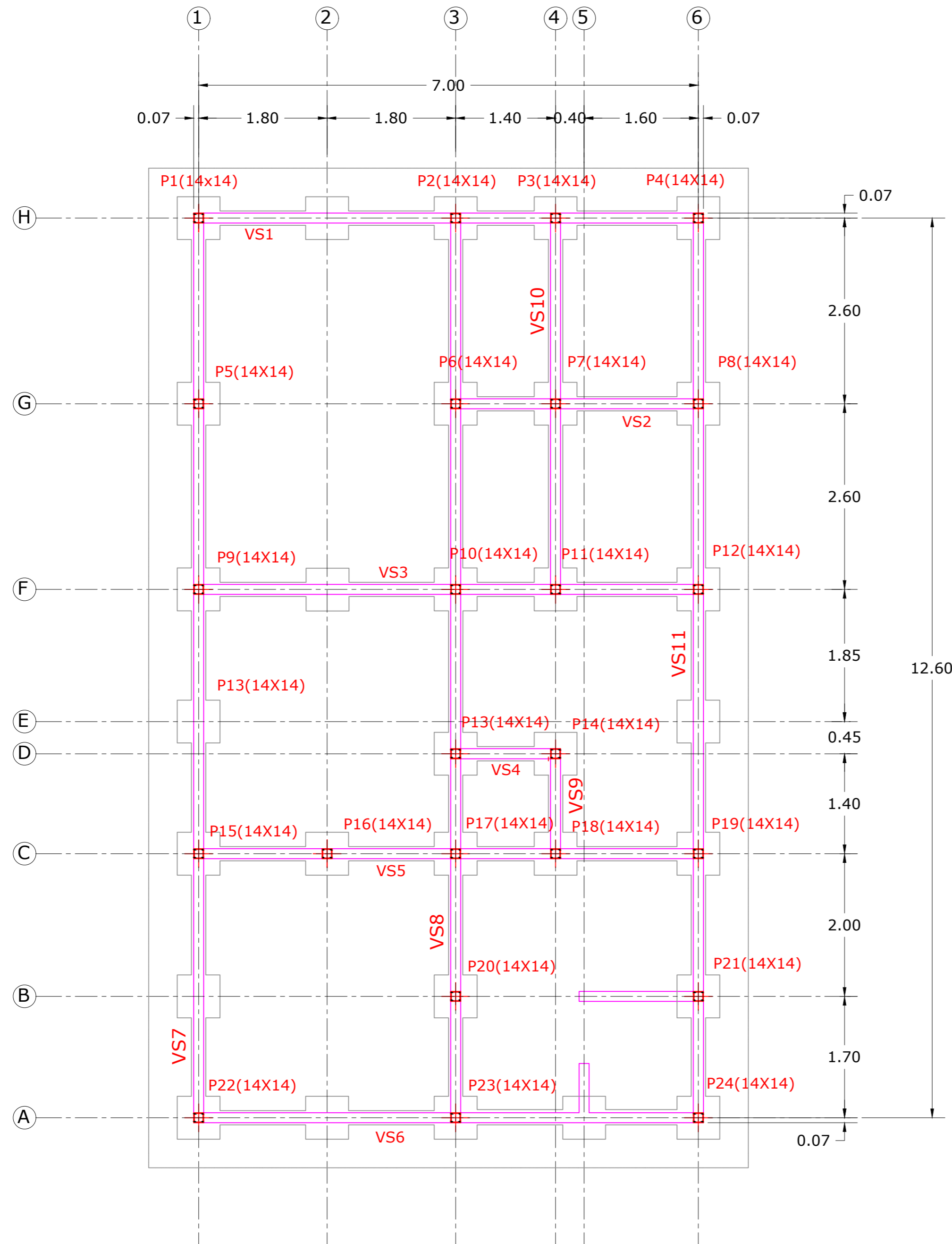
LOCAÇÃO DE PILARES / VIGAS SUPERIORES / LAJE - SETOR ADMINISTRATIVO ESC - 1:50
